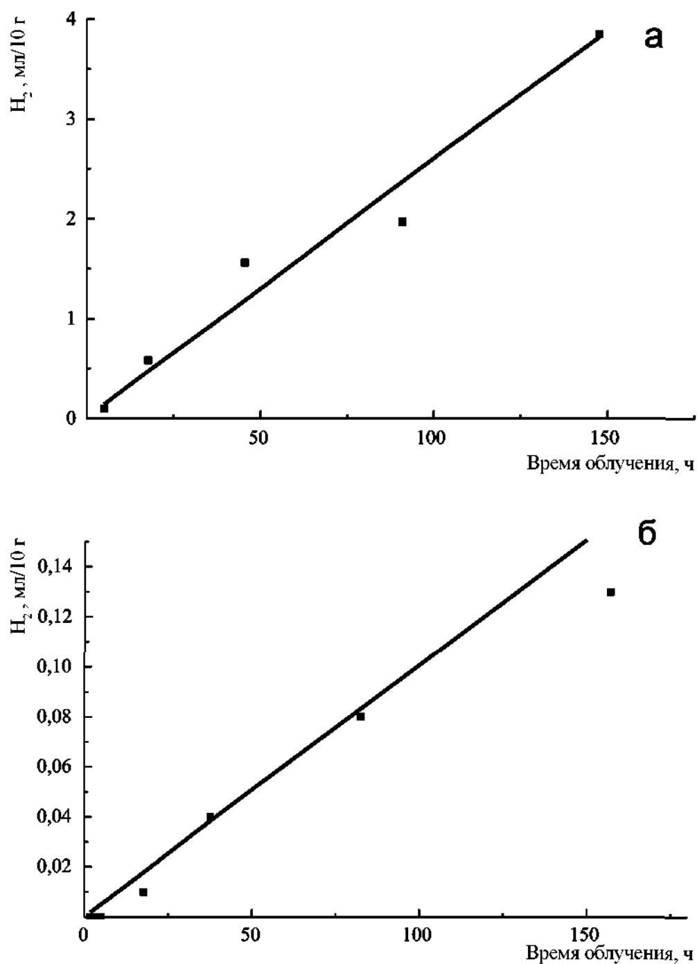
Рис. 3. Зависимость объема выделившегося H 2 от времени \gamma -облучения цементного компаунда (10 г), приготовленного на воде (27 масс. %) (а) и на водном растворе NaNO 3 (15 масс. % NaNO 3 и 25 масс. % воды) (б). Мощность дозы 5,7 кГр/ч
